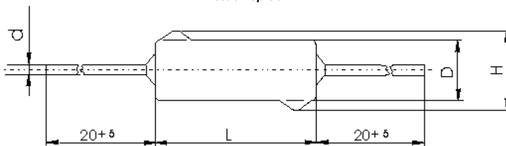
Резистор С5-42В:
