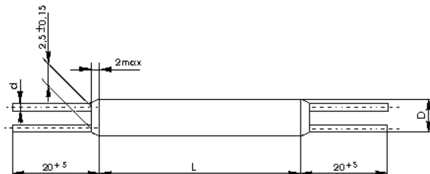
Резистор С5-42БВ:
